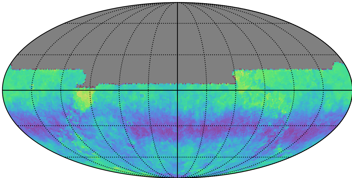
noroll_v3.4_10yrs u: Kuiper rotSkyPos
