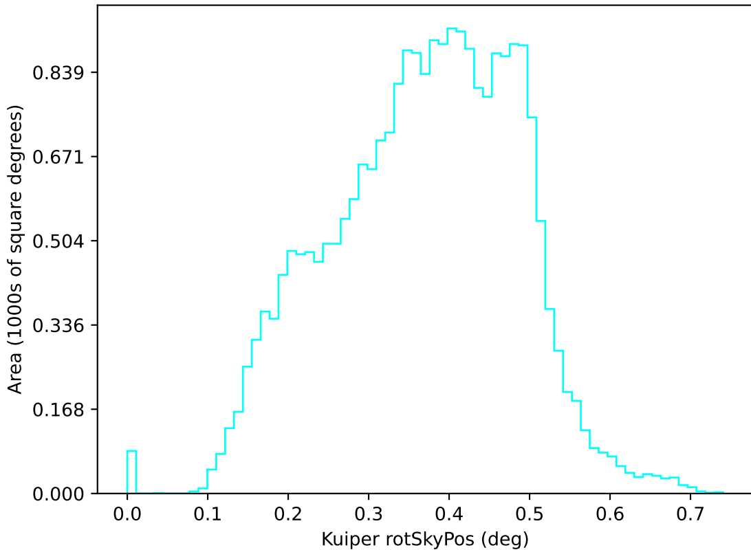
noroll_v3.4_10yrs u: Kuiper rotSkyPos
