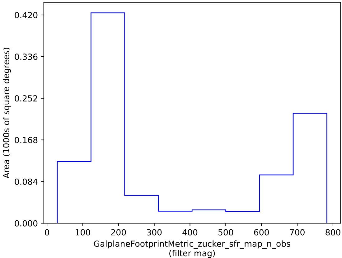
noroll_v3.4_10yrs : GalplaneFootprintMetric_zucker_sfr_map_n_obs
