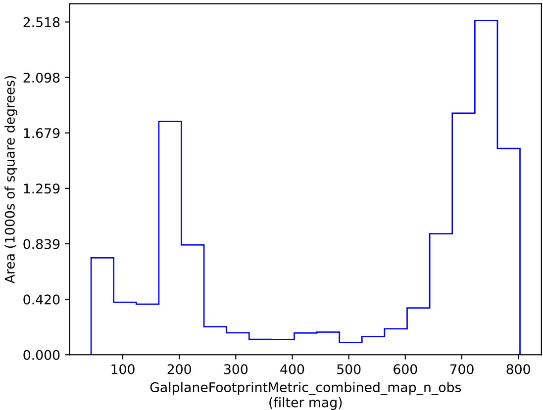
noroll_v3.4_10yrs : GalplaneFootprintMetric_combined_map_n_obs
