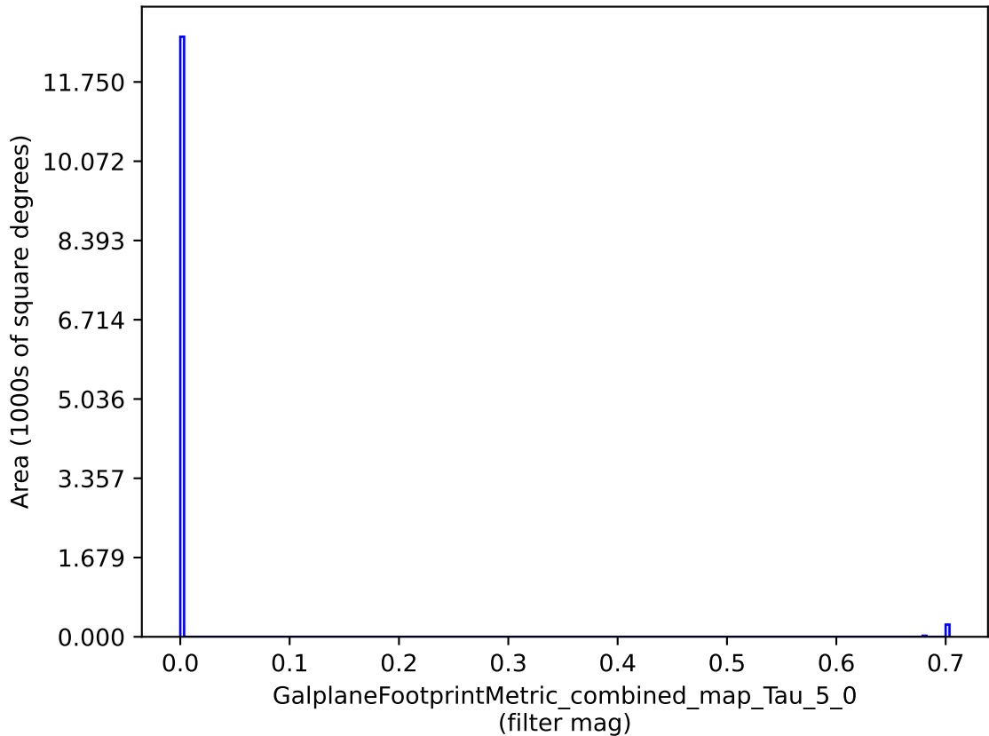
noroll_v3.4_10yrs : GalplaneFootprintMetric_combined_map_Tau_5_0
