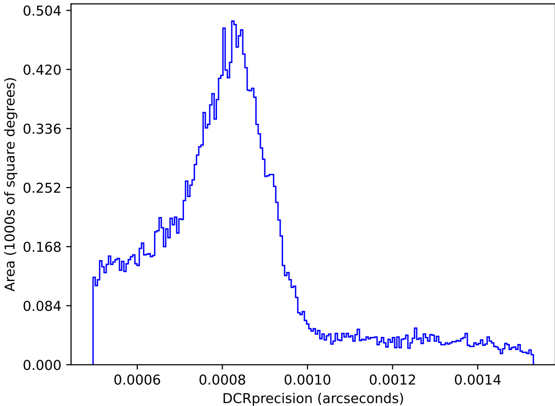
noroll_v3.4_10yrs : DCRprecision
