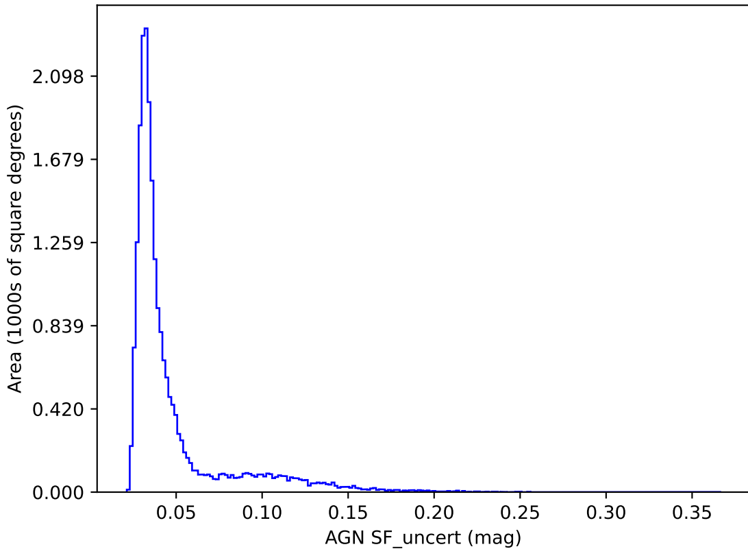
noroll_v3.4_10yrs y band: AGN SF_uncert
