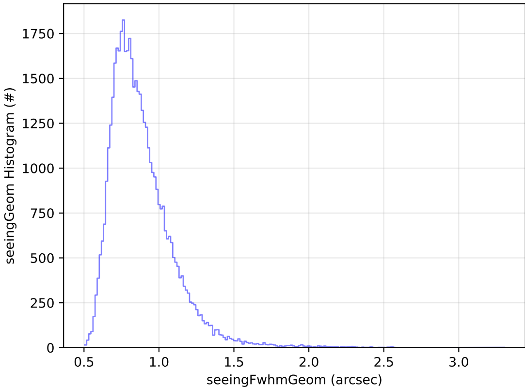
noroll_v3.4_10yrs Yr 1 y band: seeingGeom Histogram
