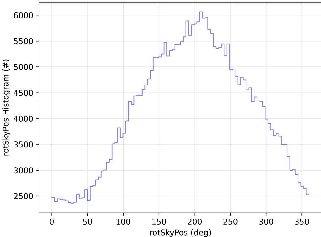
noroll_v3.4_10yrs WFD y band: rotSkyPos Histogram
