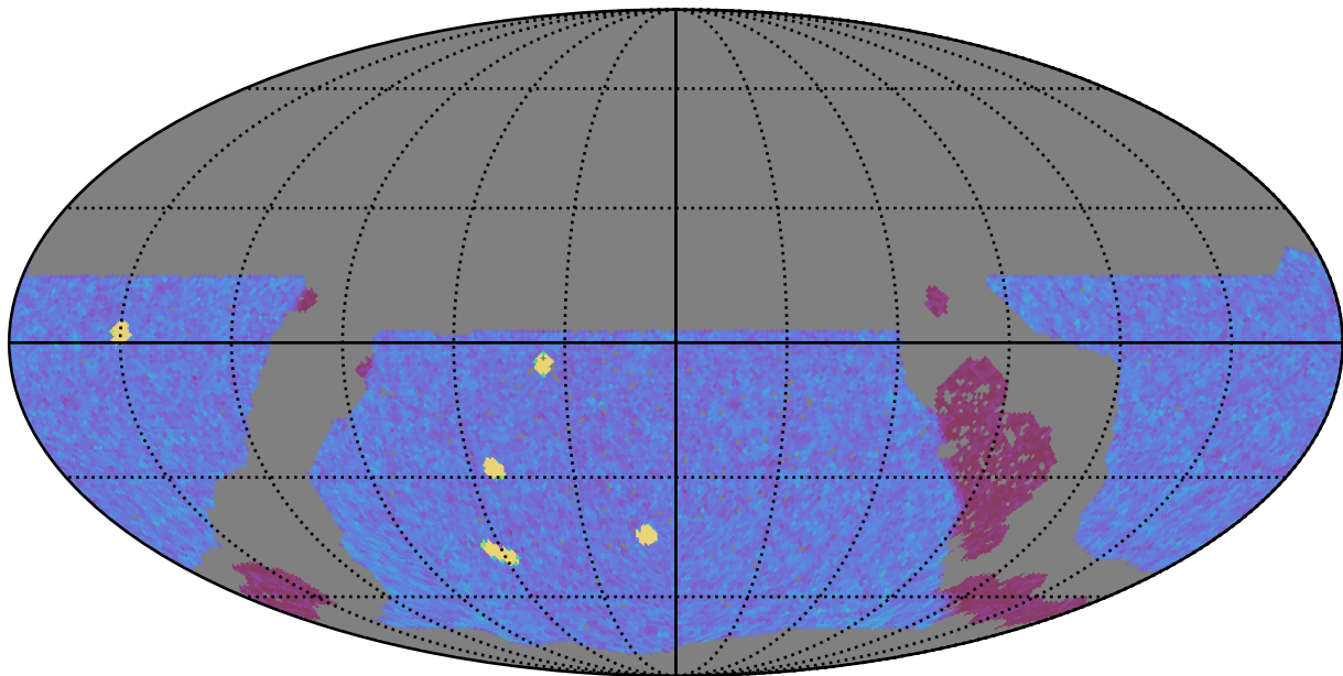
noroll_v3.4_10yrs WFD y band: NVisits
