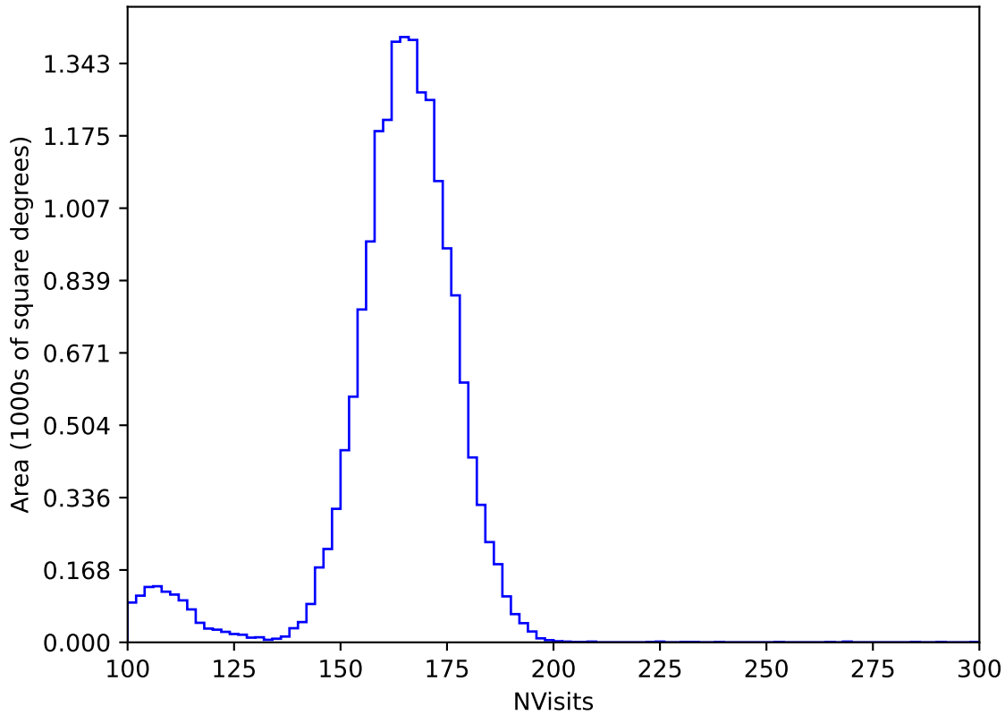
noroll_v3.4_10yrs WFD y band: NVisits
