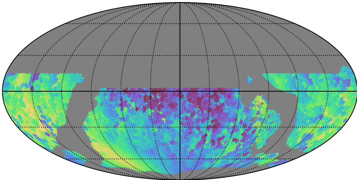
noroll_v3.4_10yrs WFD y band: Min solarElong
