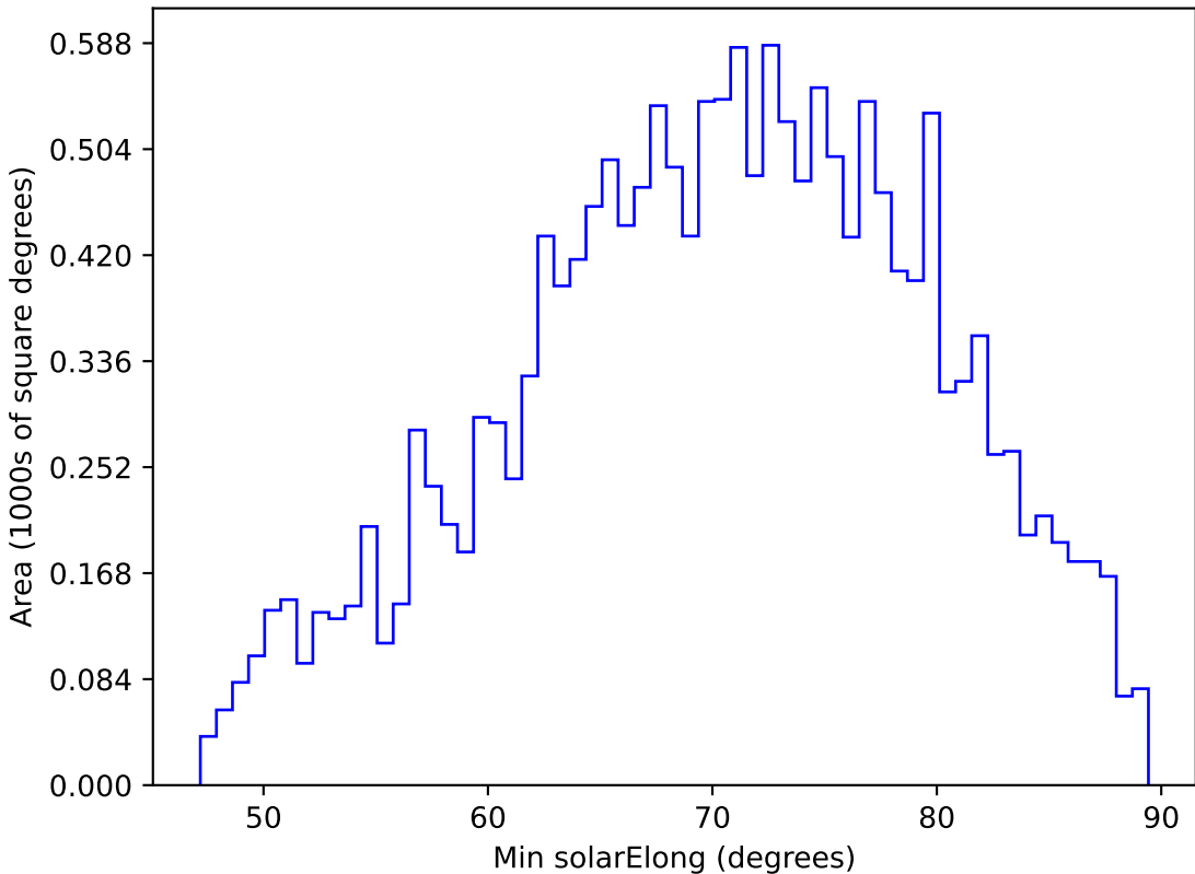
noroll_v3.4_10yrs WFD y band: Min solarElong
