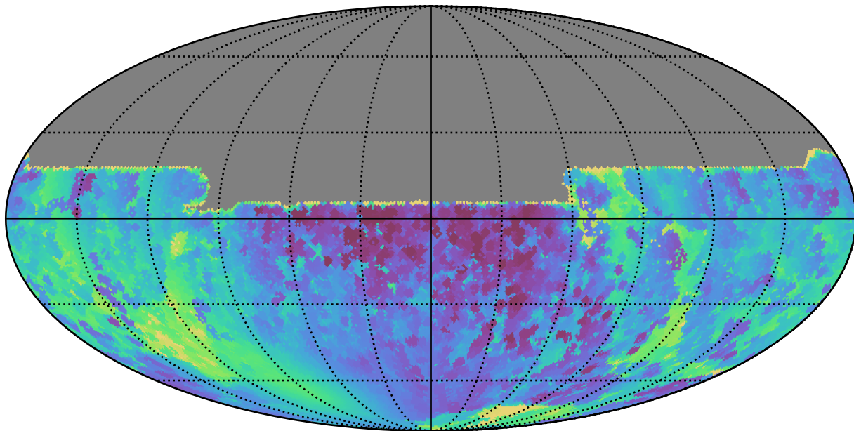
noroll_v3.4_10yrs All sky y band: Min solarElong
