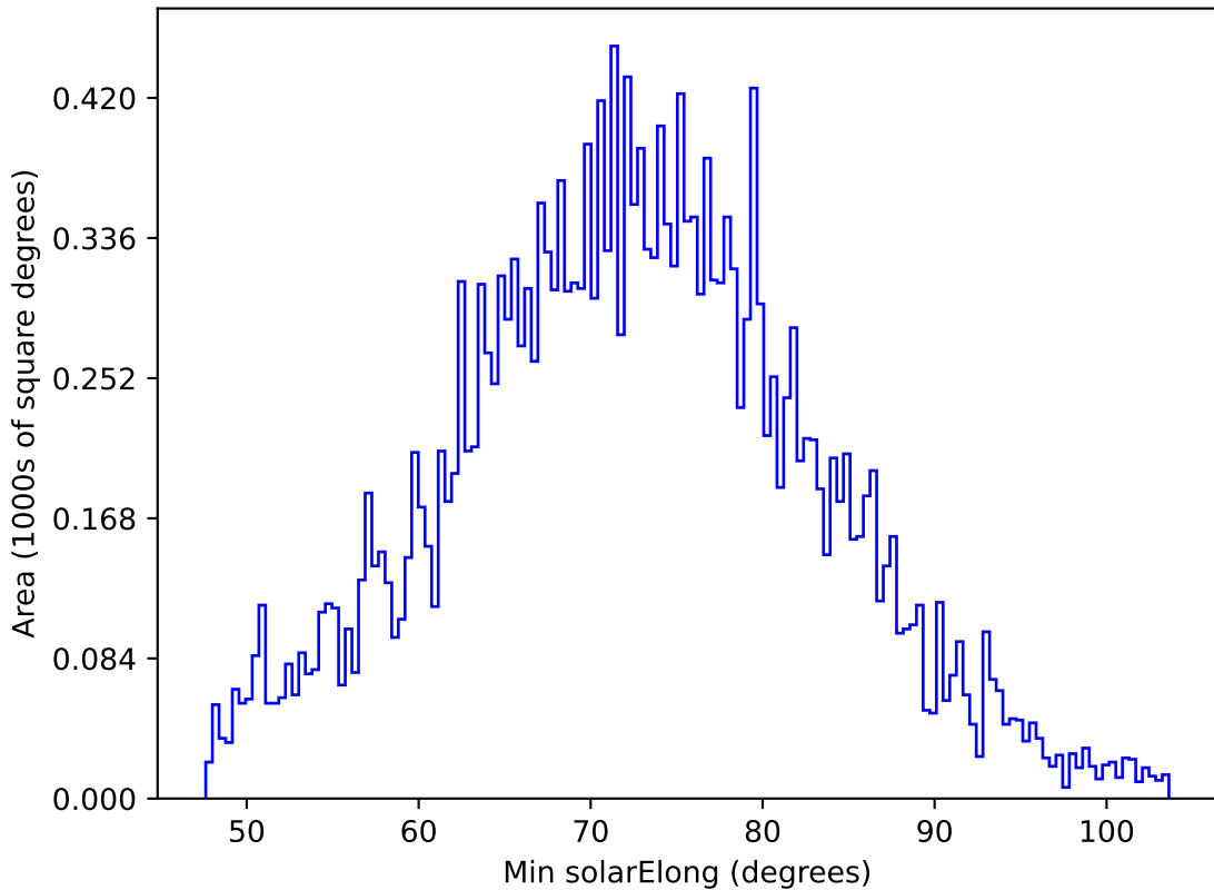
noroll_v3.4_10yrs All sky y band: Min solarElong
