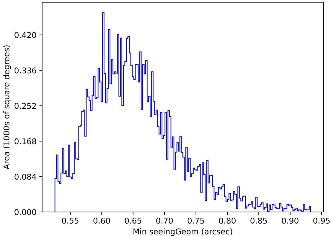
noroll_v3.4_10yrs Yr 1 y band: Min seeingGeom
