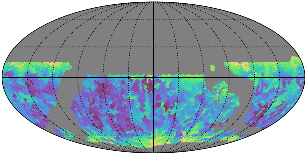
noroll_v3.4_10yrs WFD y band: Min seeingEff
