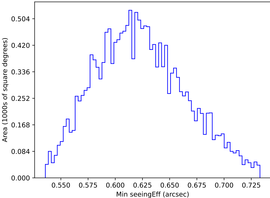
noroll_v3.4_10yrs WFD y band: Min seeingEff
