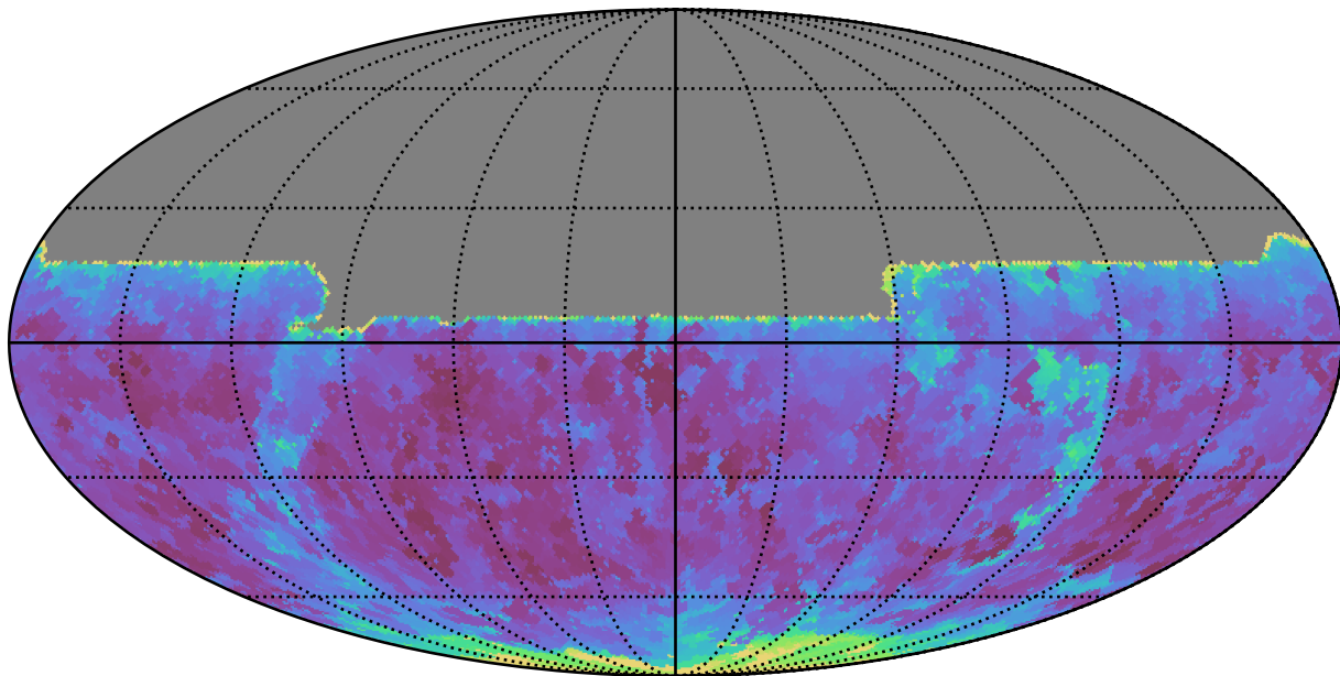
noroll_v3.4_10yrs All sky y band: Min seeingEff
