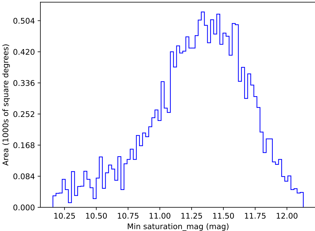
noroll_v3.4_10yrs WFD y band: Min saturation_mag
