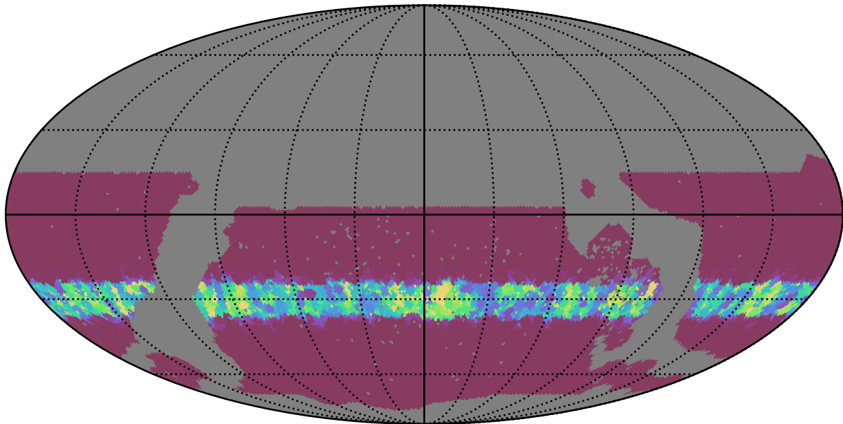
noroll_v3.4_10yrs WFD z band: Min normairmass
