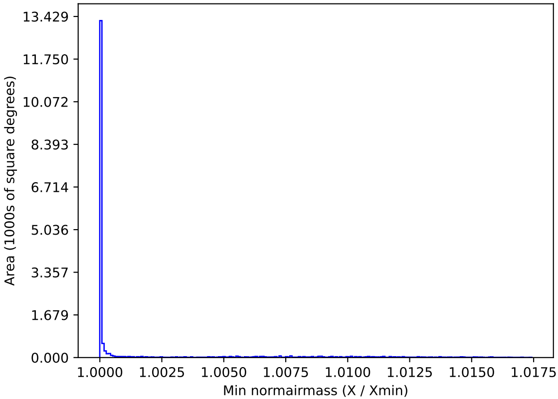
noroll_v3.4_10yrs WFD z band: Min normairmass
