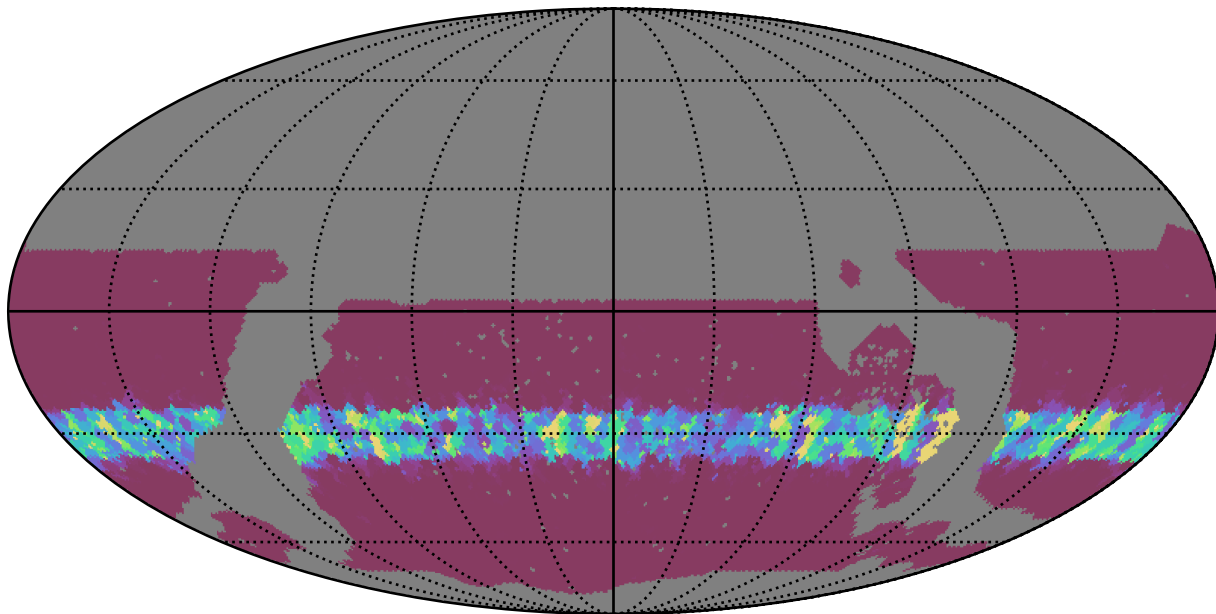
noroll_v3.4_10yrs WFD y band: Min normairmass
