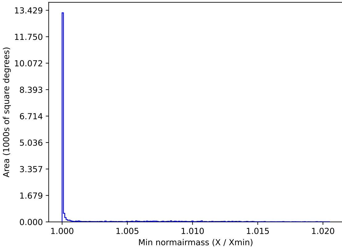
noroll_v3.4_10yrs WFD y band: Min normairmass
