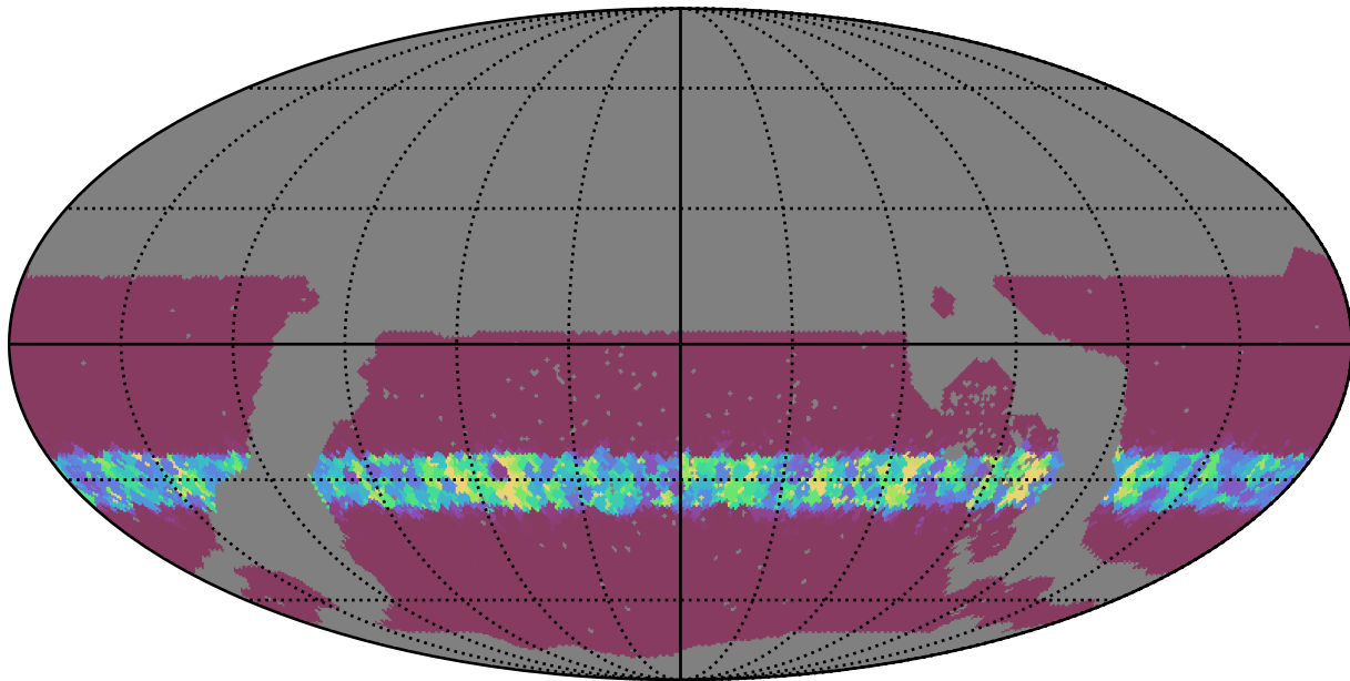
noroll_v3.4_10yrs WFD i band: Min normairmass
