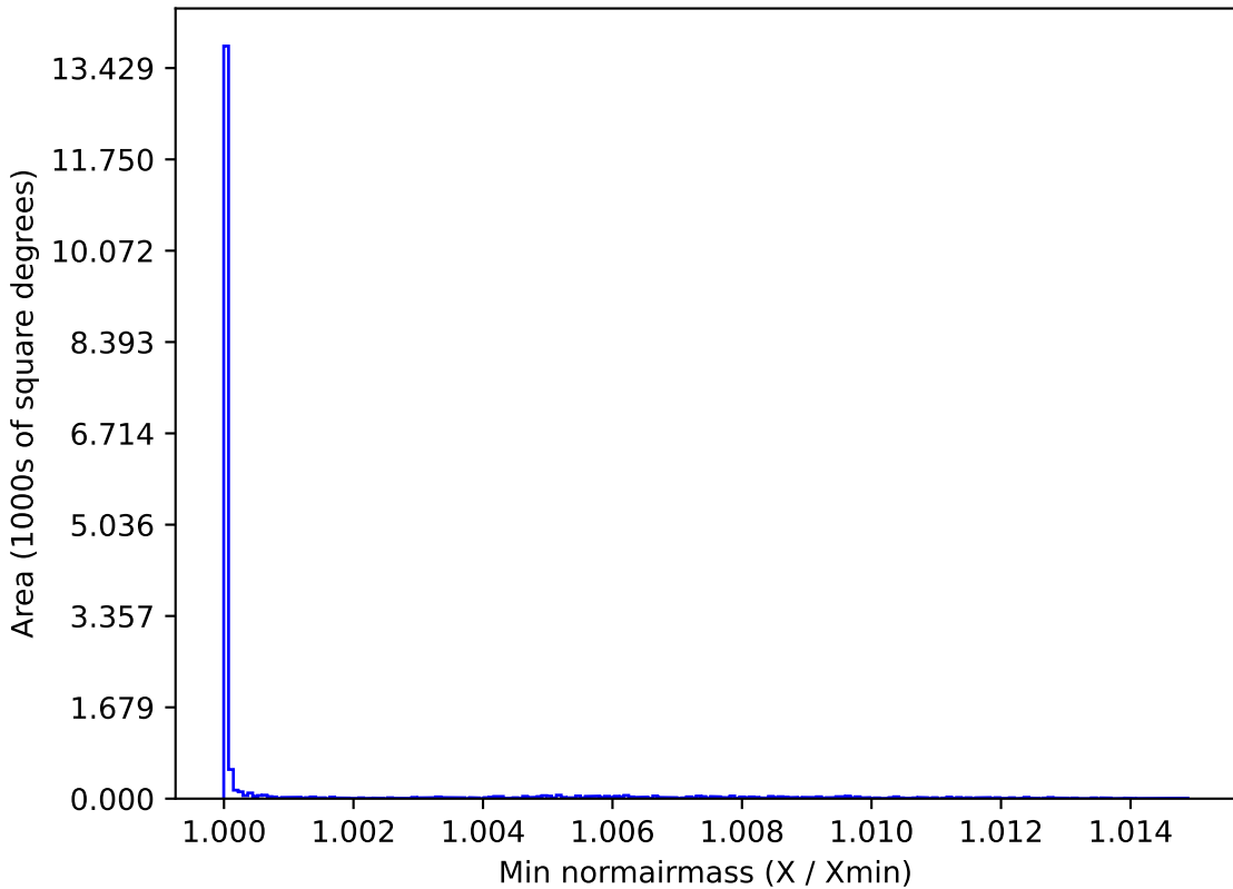
noroll_v3.4_10yrs WFD i band: Min normairmass
