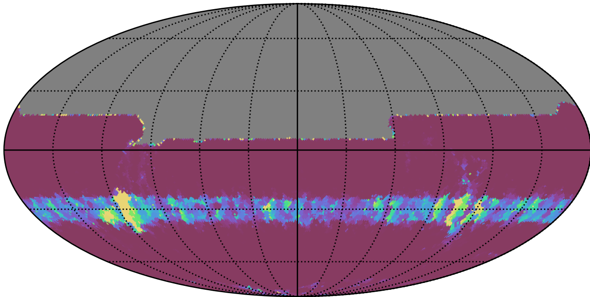
noroll_v3.4_10yrs All sky y band: Min normairmass
