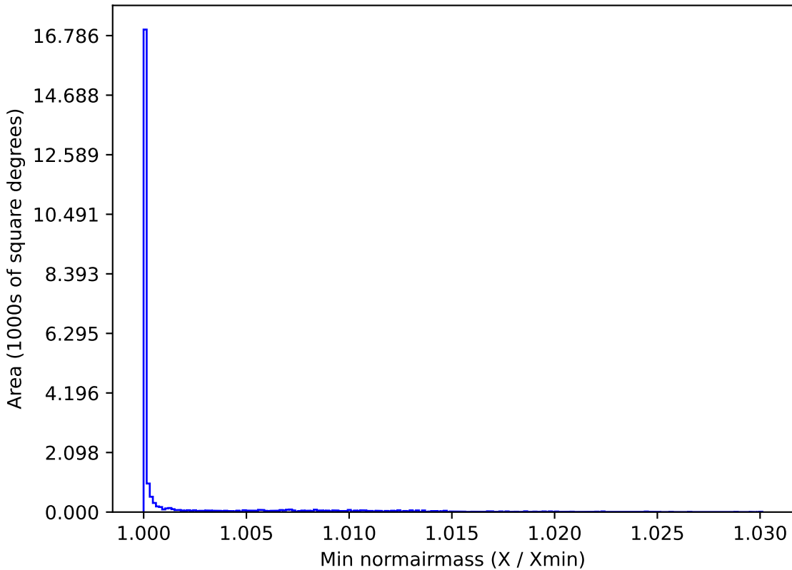
noroll_v3.4_10yrs All sky y band: Min normairmass
