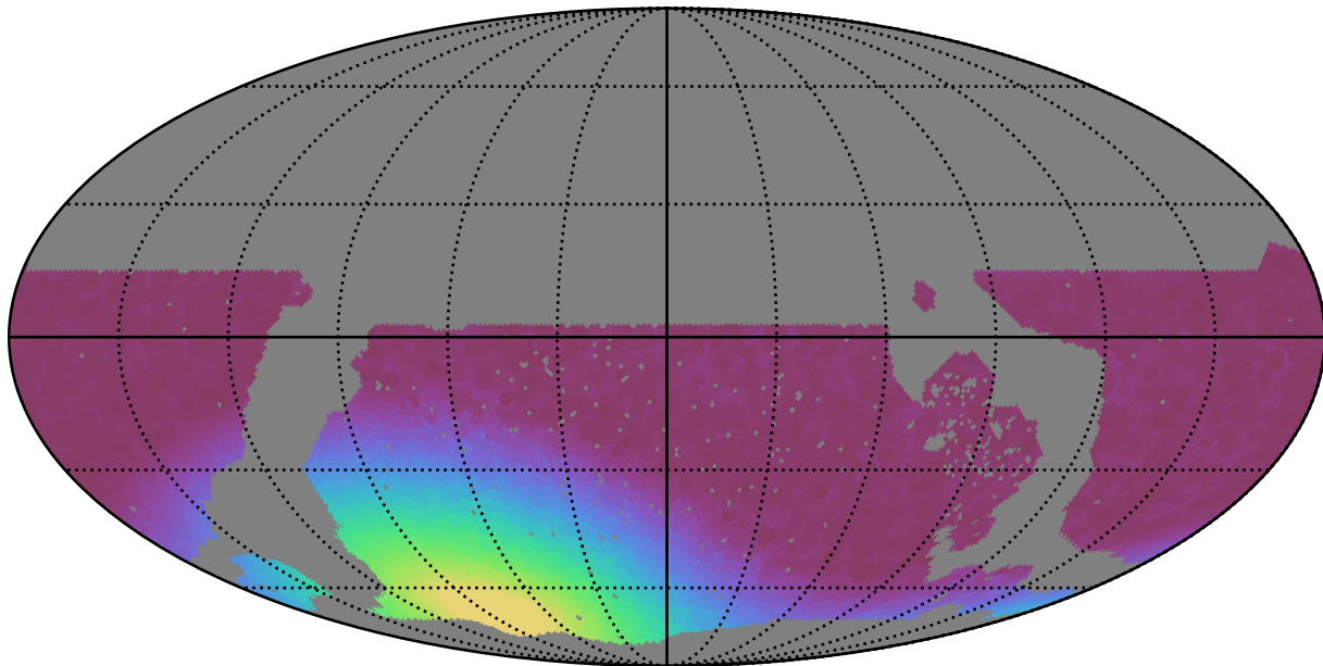
noroll_v3.4_10yrs WFD y band: Min moonDistance
