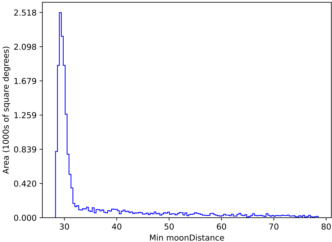
noroll_v3.4_10yrs WFD y band: Min moonDistance
