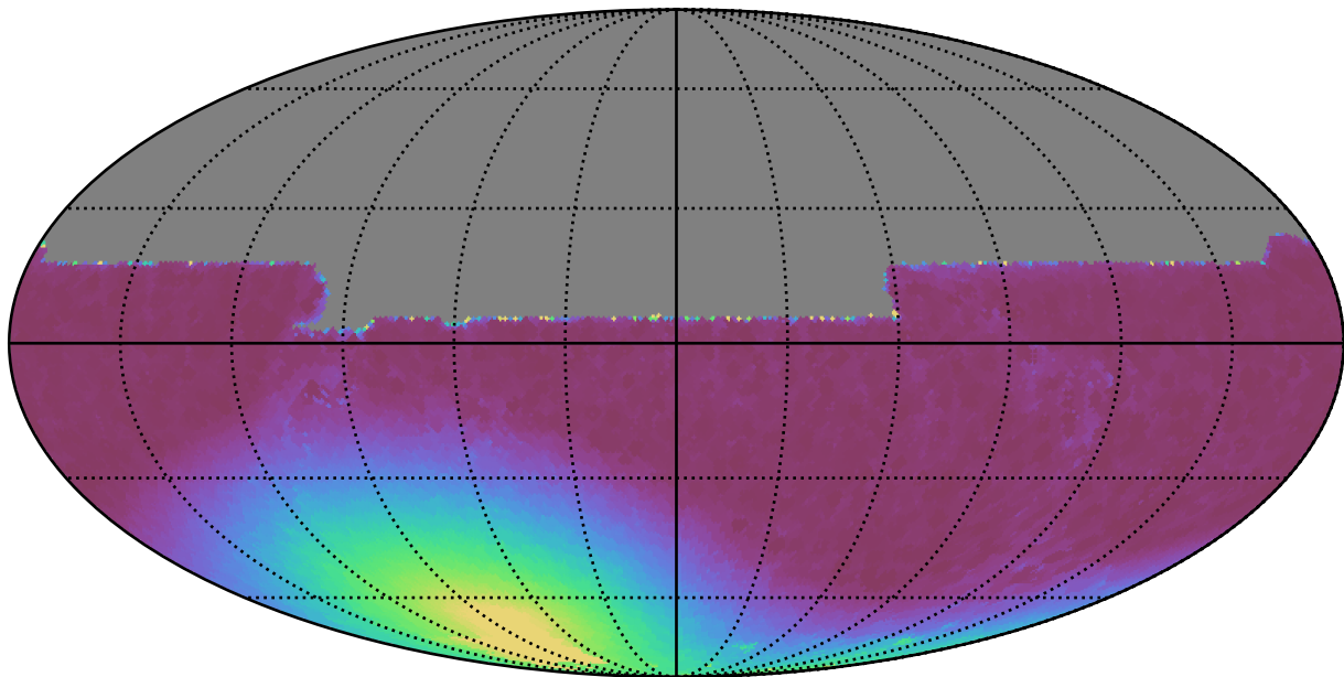
noroll_v3.4_10yrs All sky y band: Min moonDistance
