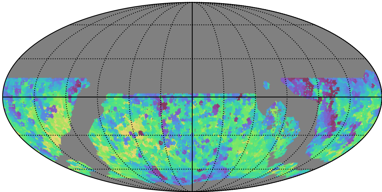
noroll_v3.4_10yrs WFD y band: Min fiveSigmaDepth
