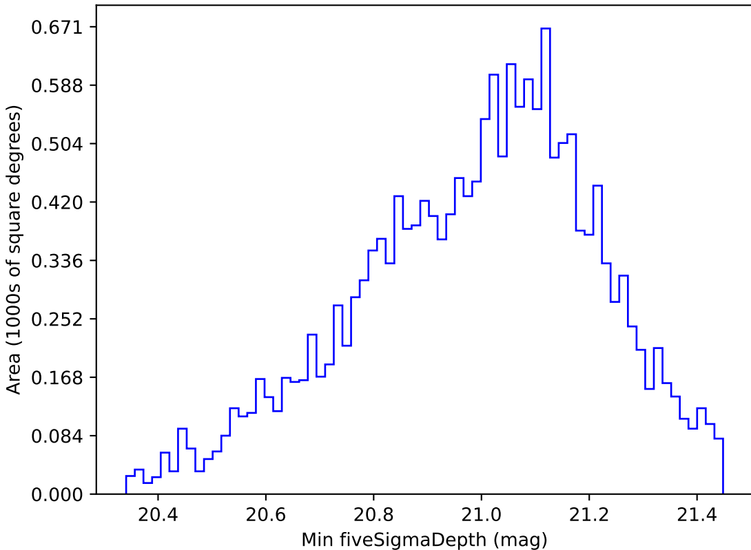
noroll_v3.4_10yrs WFD y band: Min fiveSigmaDepth
