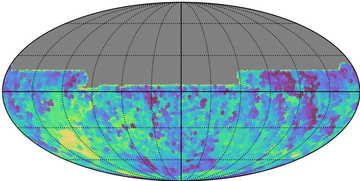
noroll_v3.4_10yrs All sky y band: Min fiveSigmaDepth
