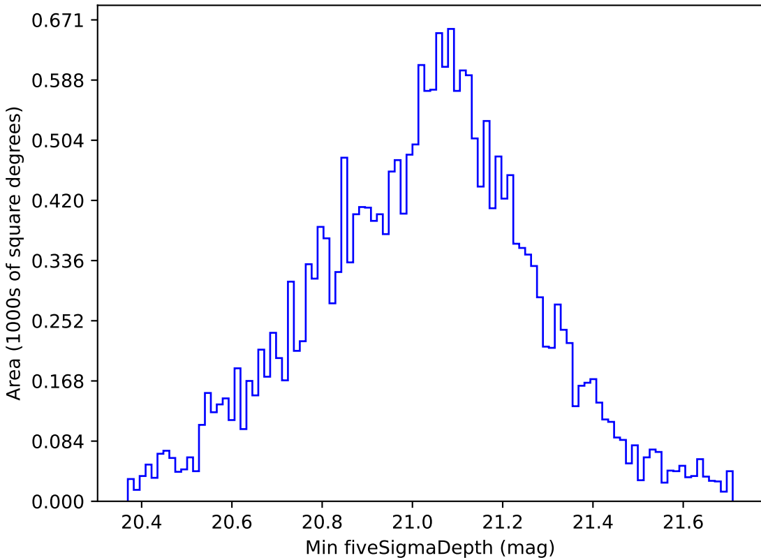
noroll_v3.4_10yrs All sky y band: Min fiveSigmaDepth
