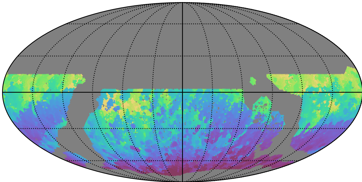
noroll_v3.4_10yrs WFD z band: Min HA
