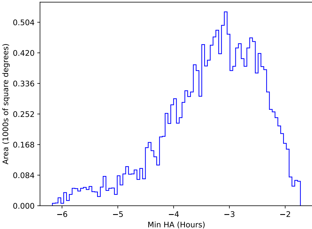
noroll_v3.4_10yrs WFD y band: Min HA
