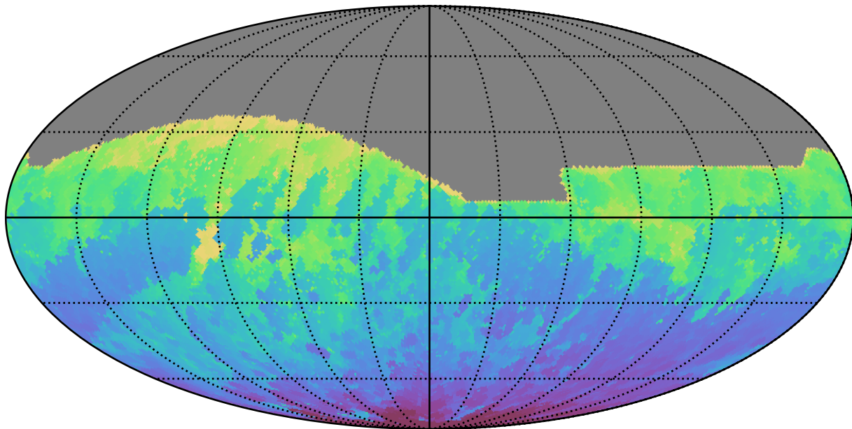
noroll_v3.4_10yrs All sky z band: Min HA
