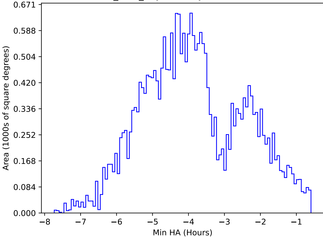
noroll_v3.4_10yrs All sky z band: Min HA
