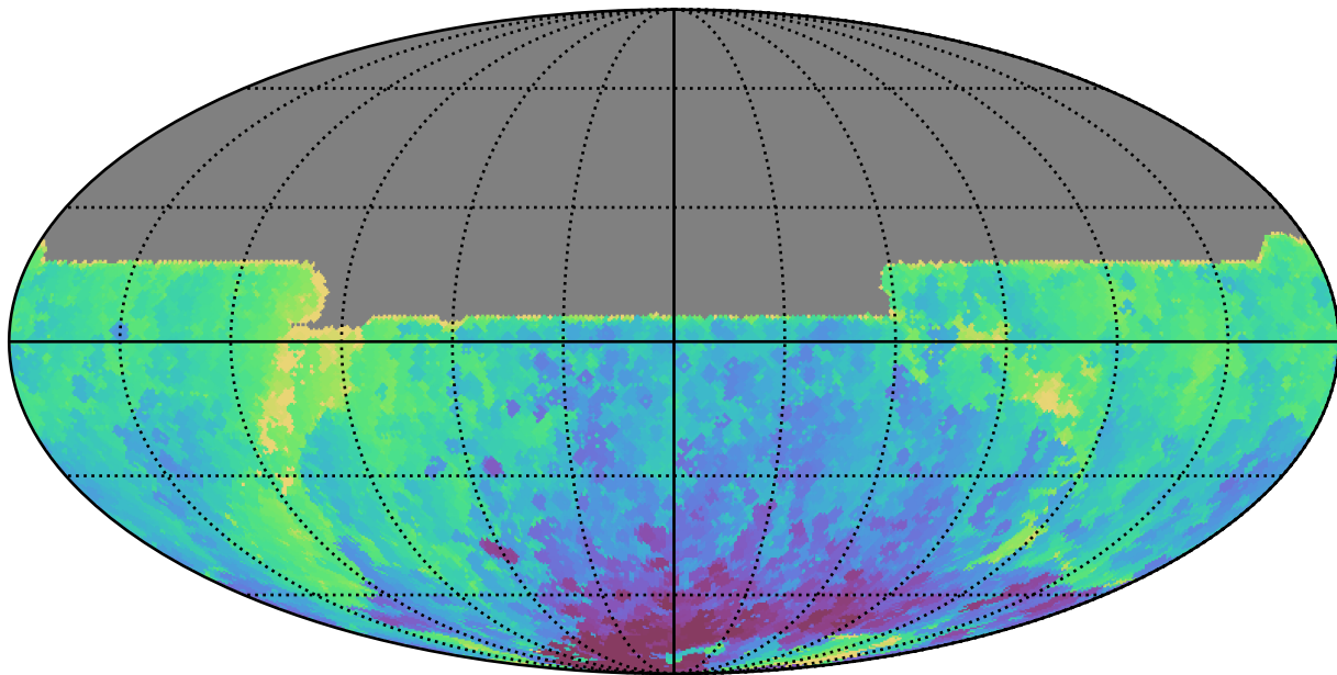
noroll_v3.4_10yrs All sky y band: Min HA
