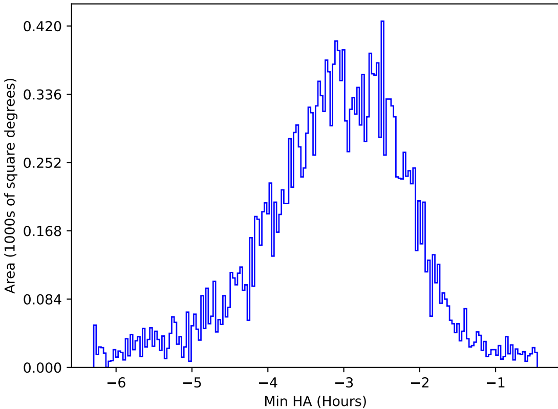
noroll_v3.4_10yrs All sky y band: Min HA
