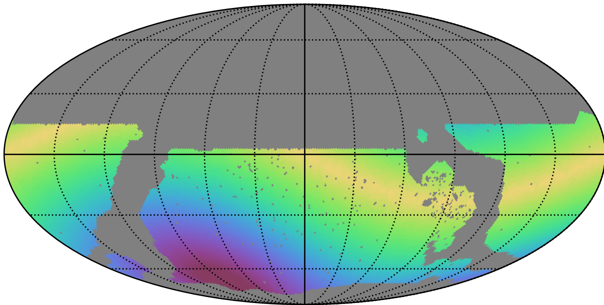
noroll_v3.4_10yrs WFD y band: Max solarElong
