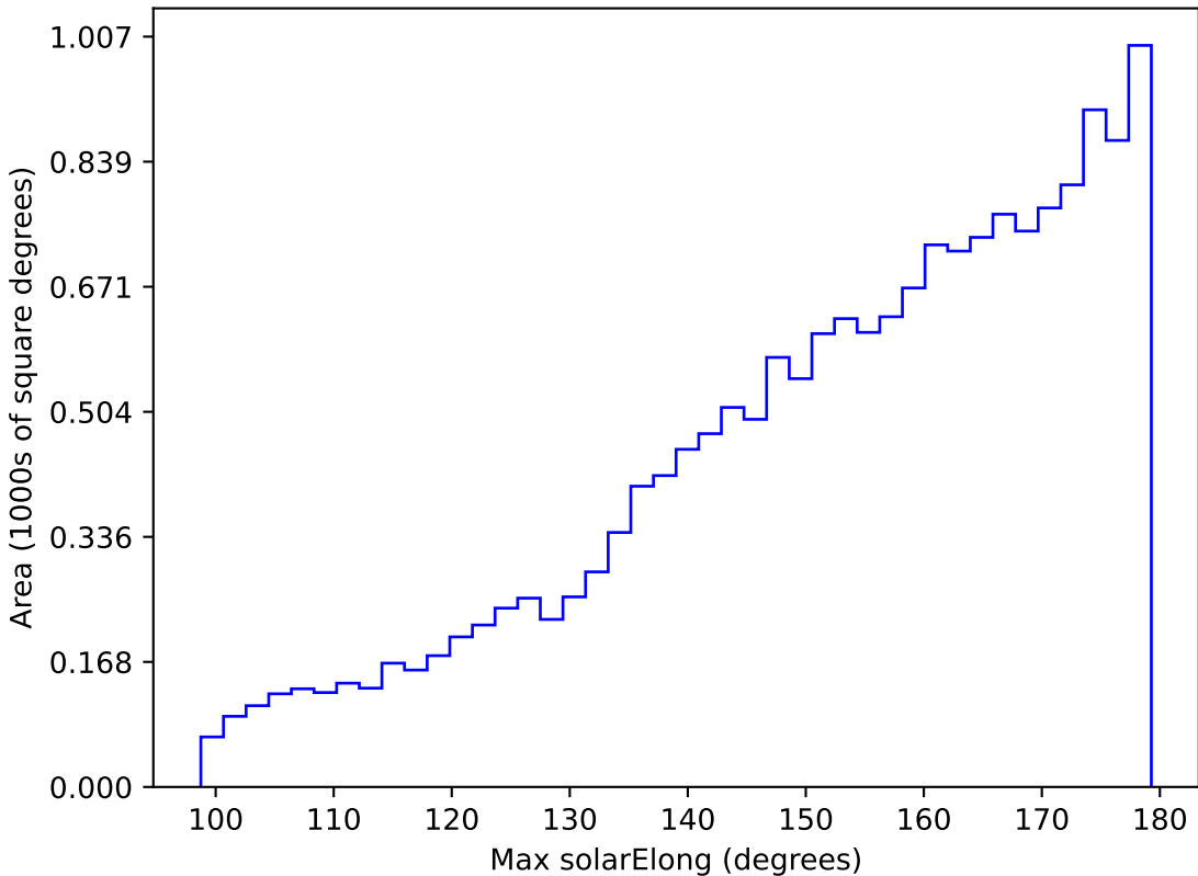
noroll_v3.4_10yrs WFD y band: Max solarElong
