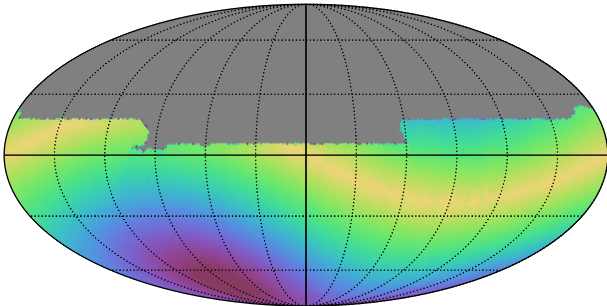
noroll_v3.4_10yrs All sky y band: Max solarElong
