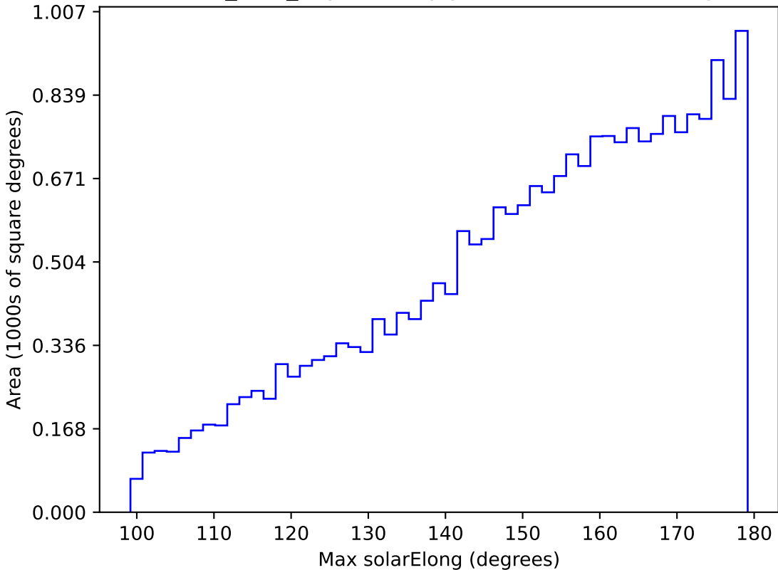
noroll_v3.4_10yrs All sky y band: Max solarElong
