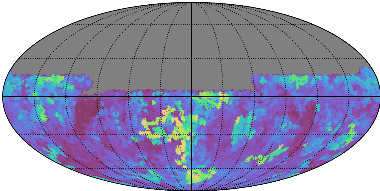
noroll_v3.4_10yrs Yr 1 y band: Max seeingGeom
