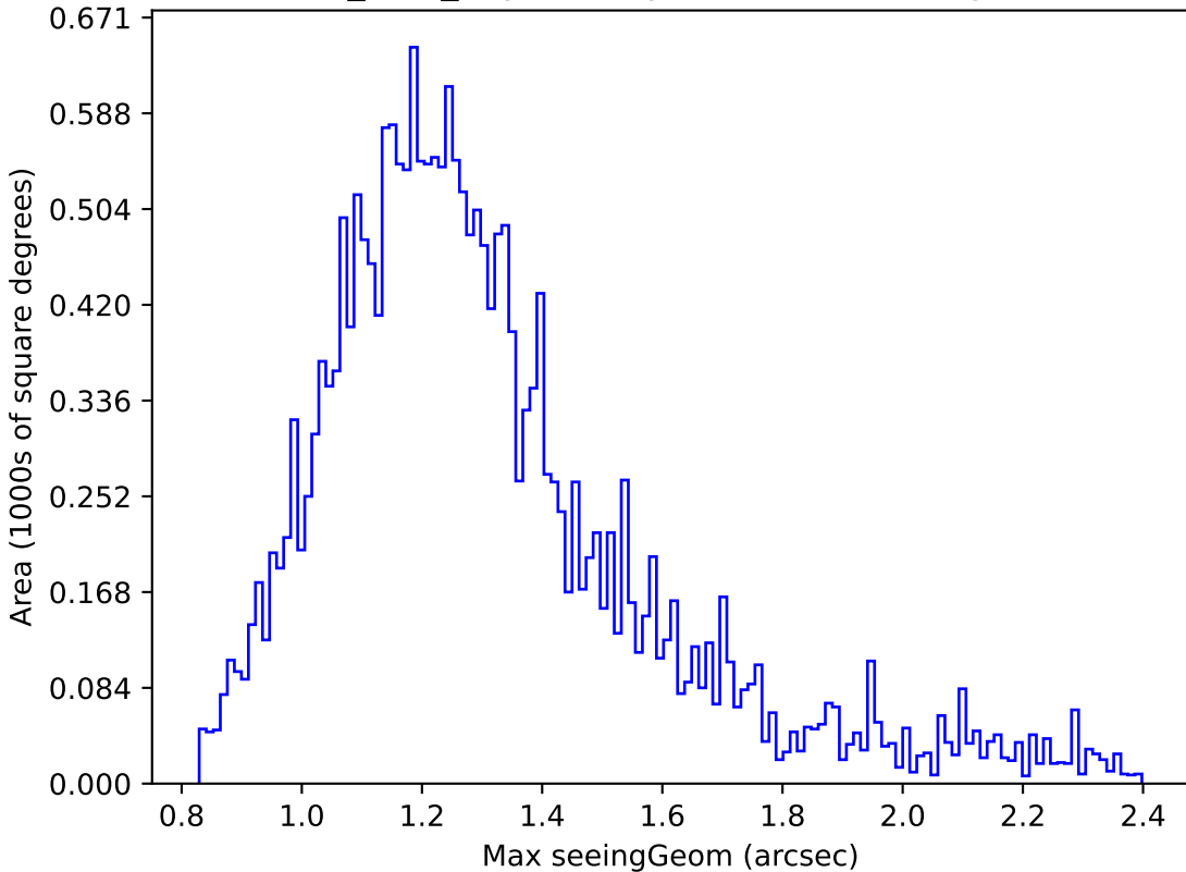
noroll_v3.4_10yrs Yr 1 y band: Max seeingGeom
