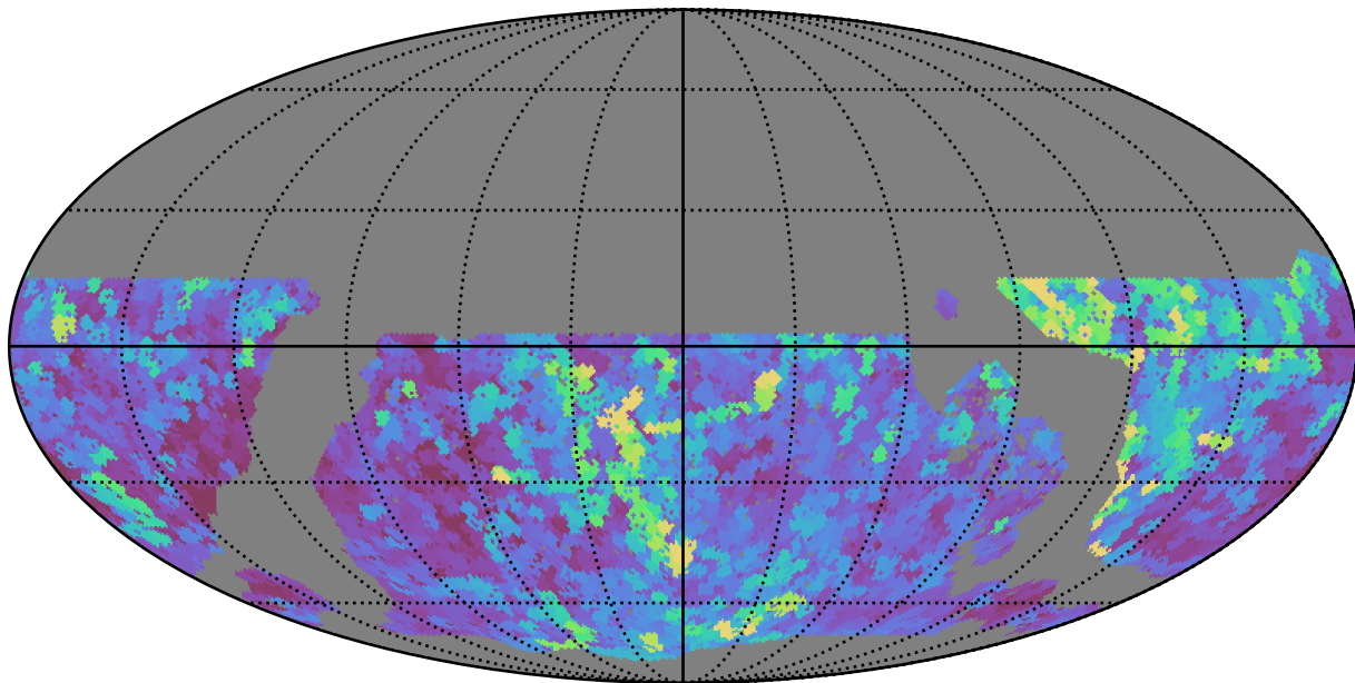
noroll_v3.4_10yrs WFD y band: Max seeingEff
