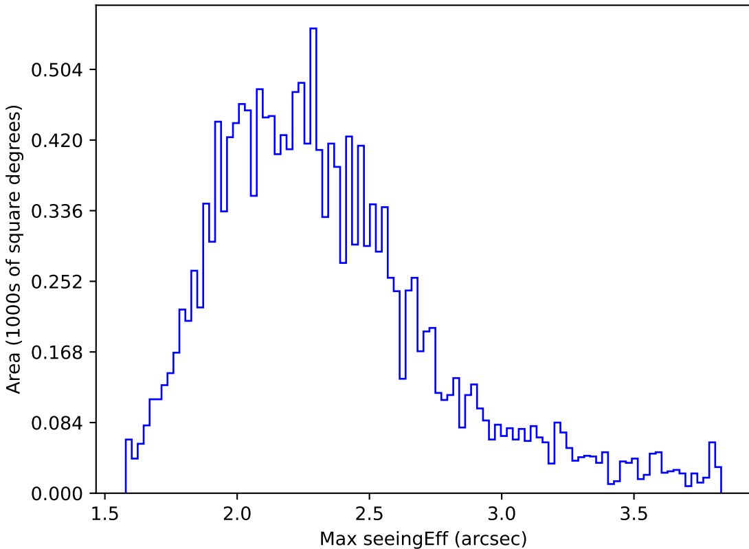
noroll_v3.4_10yrs WFD y band: Max seeingEff
