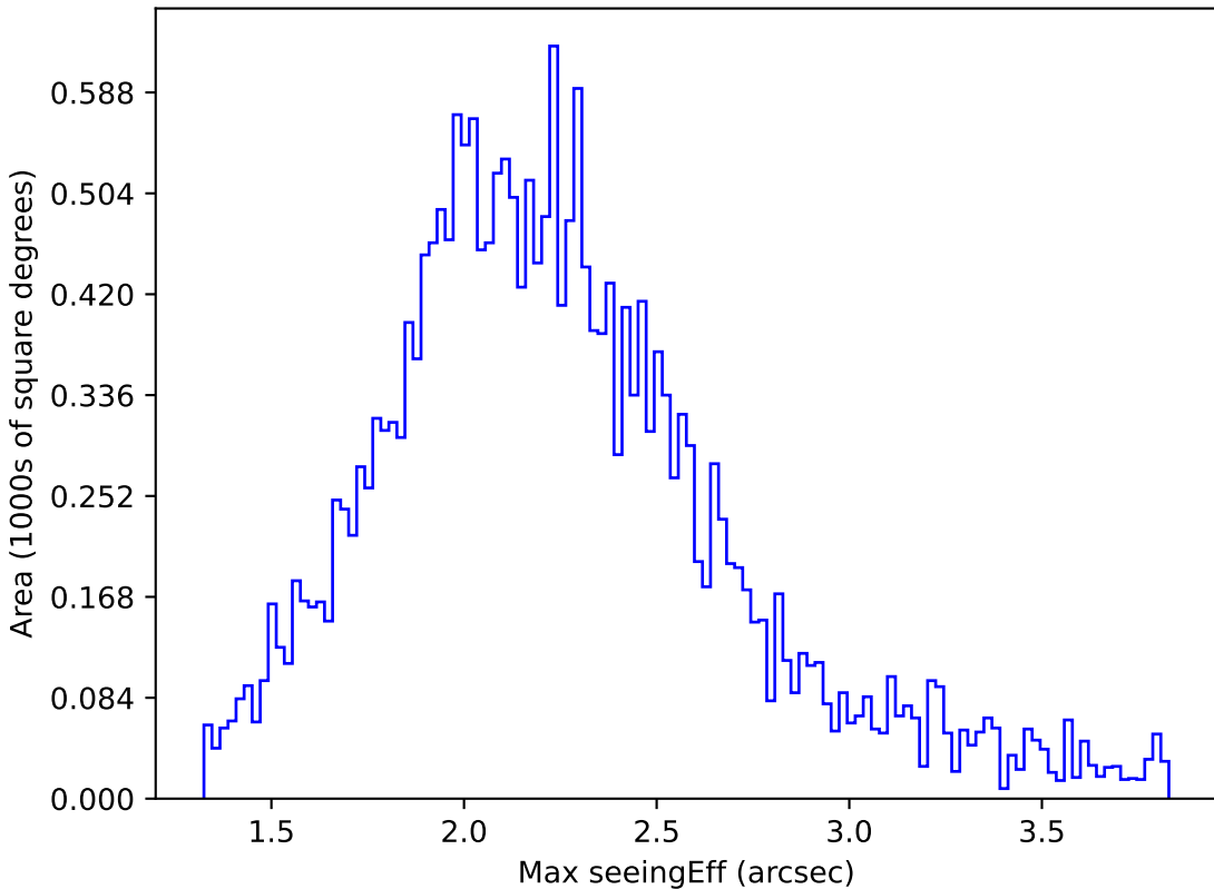
noroll_v3.4_10yrs All sky y band: Max seeingEff
